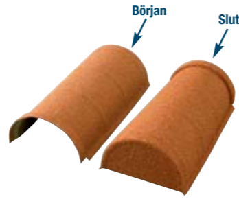
3 Decra ändnockpanna med ändbotten Start/slut. Nyttolängd 400 mm. Decra rundad nockkupa Till nock och valmnock. Nyttolängd 400 mm. 2,5 st/m.
